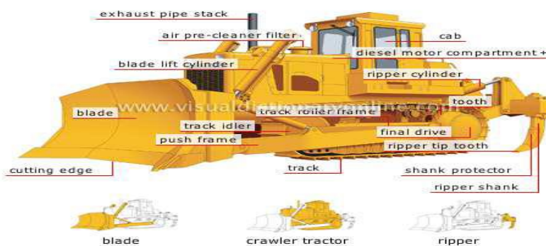
Fig. Bulldozer
