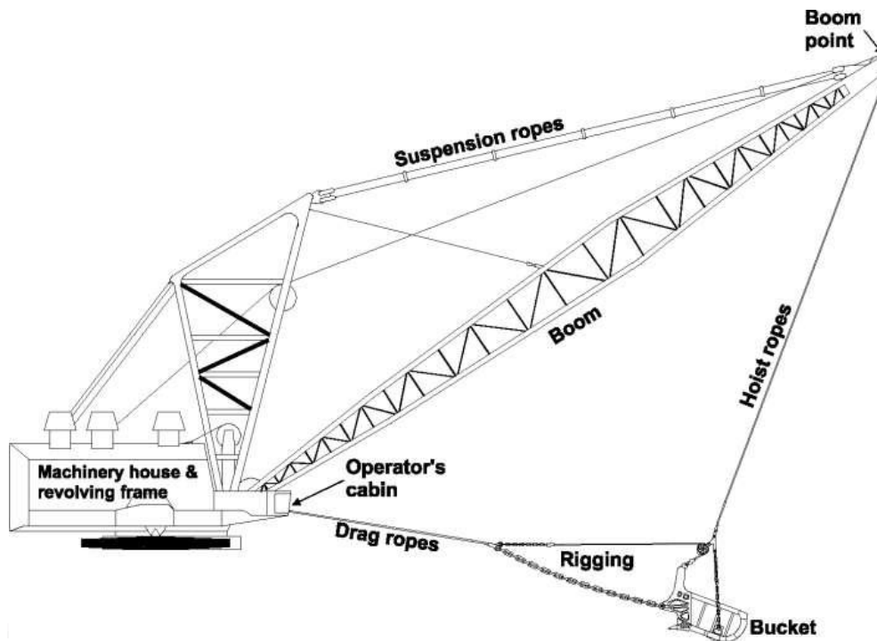
Fig. Dragline
